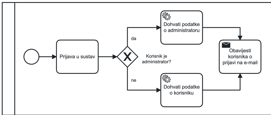
Slika 2: Nakon odabrane opcije, jednostavno proslijeđujemo tok prema sljedećoj aktivnosti
