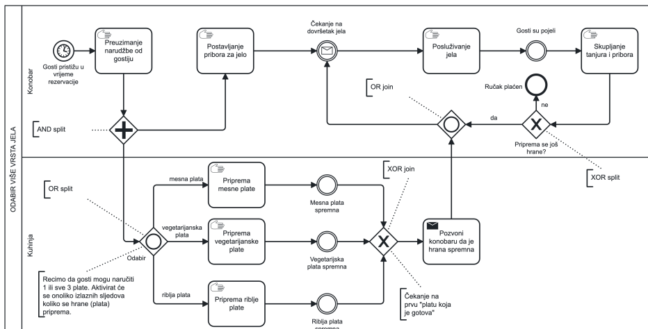
Slika 18: Proces posluživanja više vrsta jela u restoranu, modeliran na način da konobar dostavlja jela čim su spremna. Primjer pokazuje kako je moguće kombinirati različite vrste skretnica grananja i spajanja.
