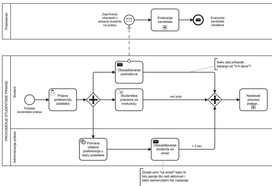
Slika 13: Proces prijave preferencija na studentsku praksu s paralelnim grananjem i spajanjem, prikazan kroz polja i staze
