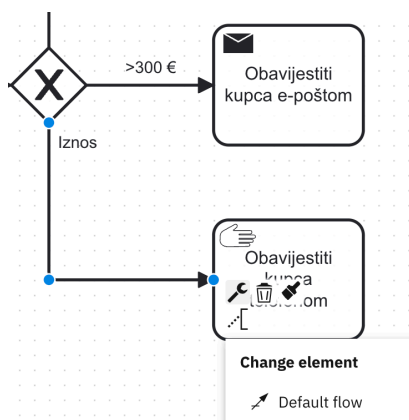
Slika 5: Odabir zadanog toka ( eng. Default flow ) iz XOR skretnice grananja. Iako je moguće definirati uvjet na zadanom toku ( < 300 \text{ €} ), preporuka je zadani tok (ako postoji) označiti bez uvjeta radi brže čitljivosti modela procesa.
