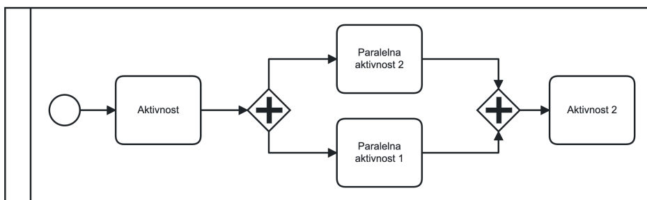
Slika 8: Ispravan način povezivanja toka nakon paralelne skretnice koristeći AND skretnicu spajanja
