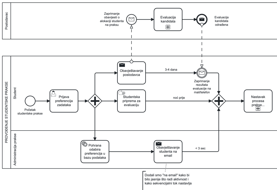
Slika 14: Proces prijave preferencija na studentsku praksu s paralelnim grananjem i spajanjem, prikazan kroz polja i staze. Uočite prijamni međudogađaj obavijesti koji označava čekanje na rezultat evaluacije poslodavca.
